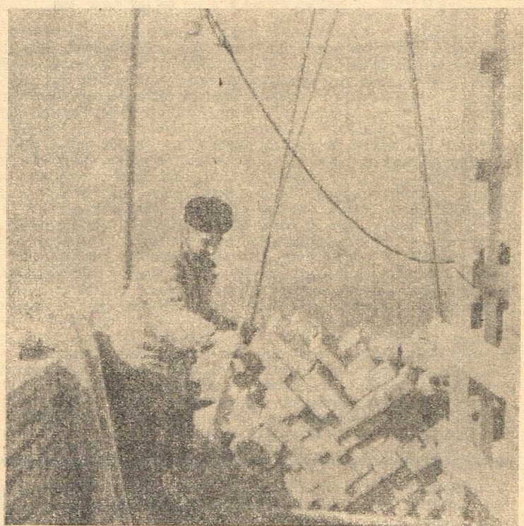
Шахта № 9—9 бис сооружается по последнему слову техники. В тресте разработан научный план строительства этого объекта. Здесь почти нет ручного труда. Механизированы все вспомогательные процессы. На снимке изображен момент приема кирпича на главном конре. Каменщики со своего рабочего места подают сигнал крановщику о том, что им нужен материал.
