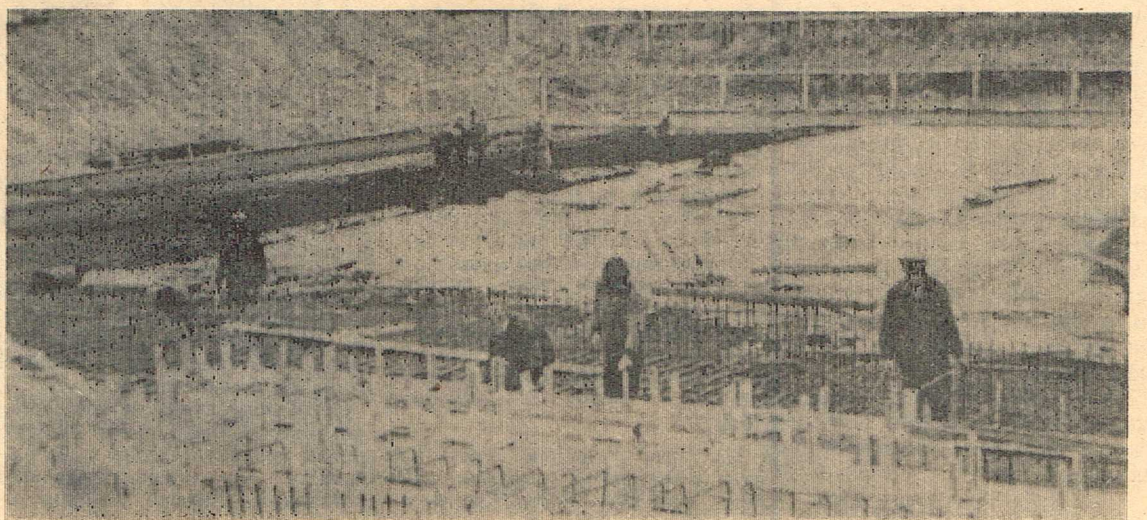
Сейчас на строительстве очистных сооружений идет установка аэротенков. Это один из наиболее важных узлов объекта, и строители пятого управления уделяют ему много внимания.
