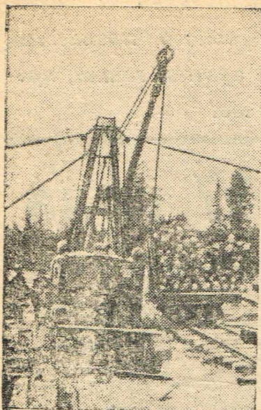
Карело-Финская ССР, Вера-дозерский механический лесопункт треста «Сев-кареллес». На снимке: механическая погрузка леса на платформы. Фото В. Поликова.
