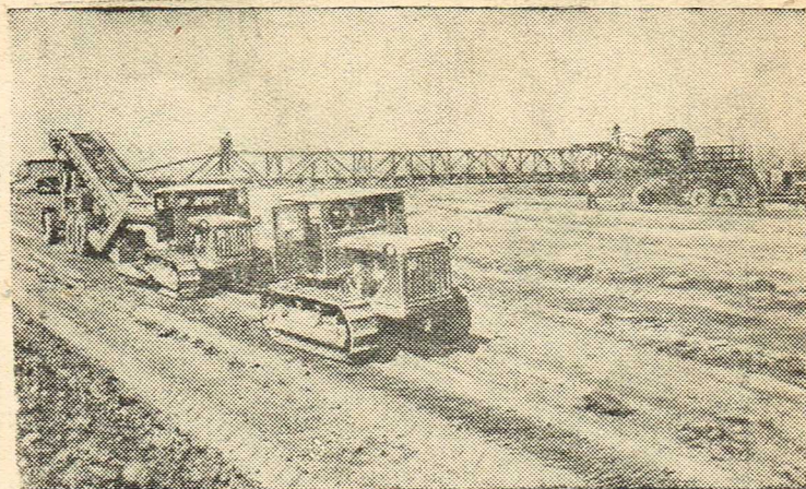
Сталинградгидрострой. На острове Зеленом начались подготовительные работы к сооружению нижнего подходного канала ш. юза. На снимке: струг за работой.
