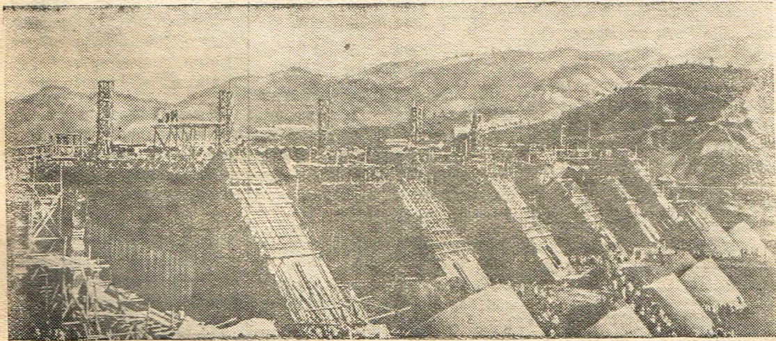
В Китайской Народной Республике для орошения полей в засушливое время года и для защиты посевов от наводнений строятся плотины, дамбы, водосбросы и каналы. На реке Бихэ в Северном Китае сооружается большое Фочзылинское водохранилище.
