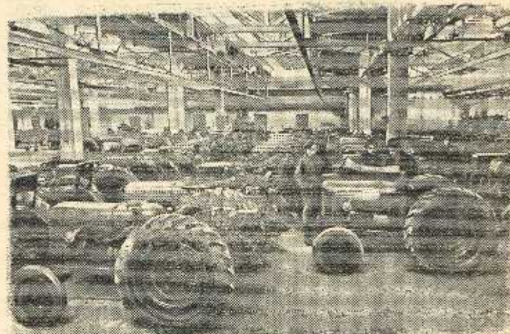
Харьков. В механосборочном корпусе тракторного завода пущен конвейер по сборке тракторов ХТЗ-7.
