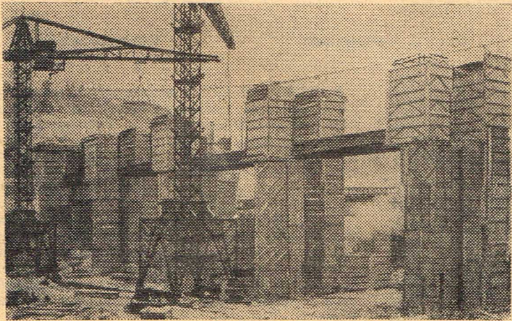
НА СНИМКЕ: вид на сооружения плотины Красноярской ГЭС в левобережном котловане.
