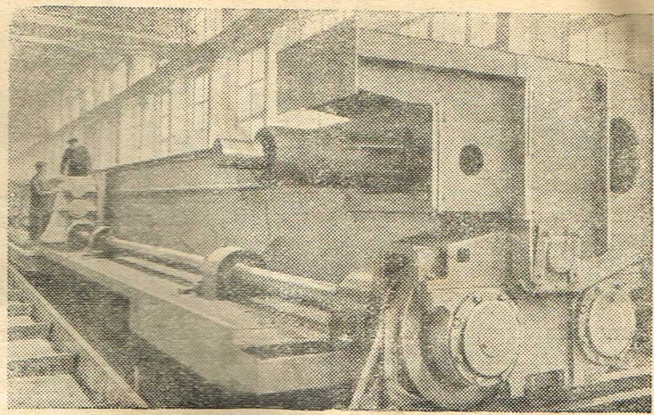
Запорожская область. Днепропетровский механический завод приступил к изготовлению стотонных мостовых кранов. На снимке: мост стотонного крана.
