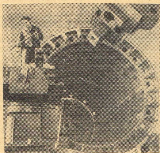
Харьков. Замечательный подарок готовит коллектив ордена Ленина завода «Электротяжмаш» имени В. И. Ленина к 100-летию со дня рождения вождя. Это уникальный турбогенератор мощностью один миллион киловатт.
