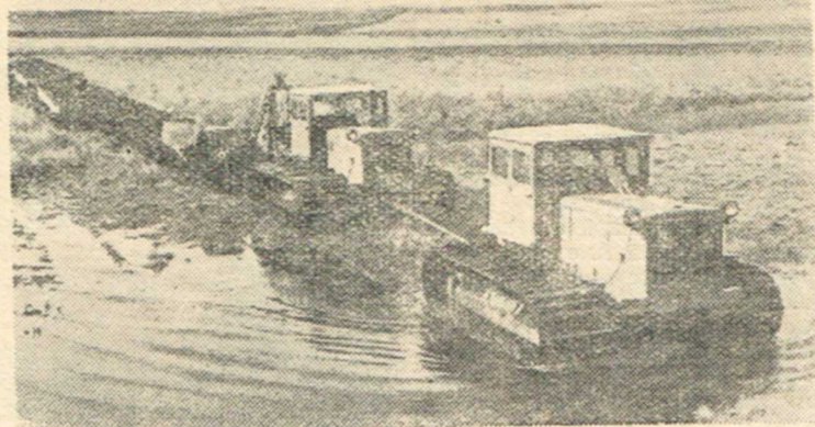
На Челябинском тракторном заводе недавно создан новый мощный болотоходный трактор «С-100Б». Он обладает проходимостью в два раза большей, чем трактор «С-80». На нем установлен дизельный двигатель в сто лошадиных сил.
