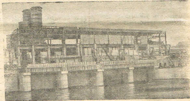
Азербайджанская ССР. Первая очередь Мингечаурской гидроэлектростанции введена в действие. Начали работать две турбины. На снимке: Мингечаурская ГЭС.
