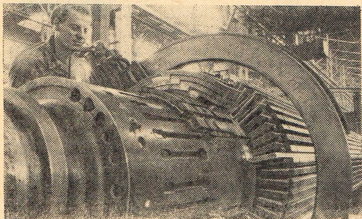
ХАРЬКОВ. На заводе «Электротяжмаш» имени В. И. Ле- нина идет изготовление крупнейшего турбогенератора. НА СНИМКЕ: ударник коммунистического труда обмот- чик турбогенераторного цеха В. Фатеев у ротора турбогенера- тора. Фото А. Татаренко. Фотохроника ТАСС.
