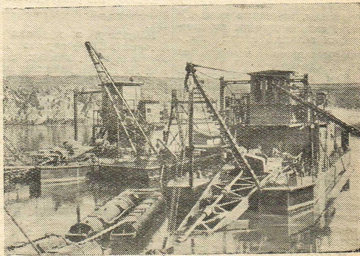
Запорожье. Бригада Щербаковского завода досрочно закончила монтаж и спустила на воду второй земснаряд, предназначенный для строительства Каховской ГЭС. На снимке: земснаряды перед отправкой в Каховку.
