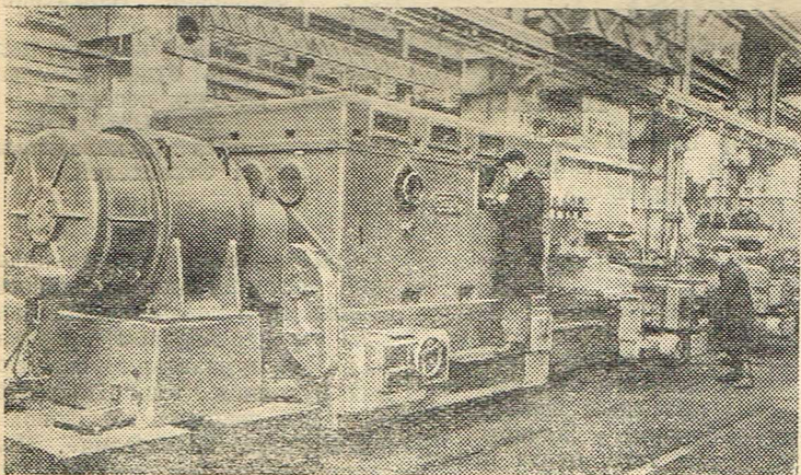
★ ★ Сталинская область. Краматорский станкостроительный завод изготавливает крупнейшие токарные станки для промышленных предприятий. Сейчас идет сборка нового тяжелого токарного станка модели «1680». Его вес—130 тонн, длина—18,5 метра. Станок предназначен для обработки деталей весом в 50 тонн.
