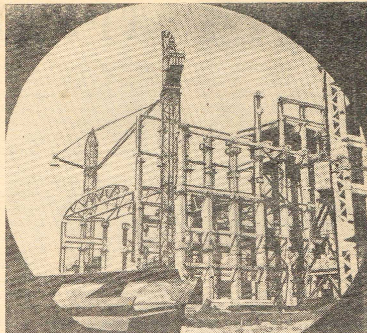
В различных районах Болгарии продолжается строительство новых и расширение существующих электроэнергетических объектов. Успешно сооружается ТЭЦ «Марина — Восток-2». Большая часть оборудования поставлена советскими предприятиями. Проектная мощность электростанции 60 тысяч киловатт. НА СНИМКЕ: строительство ТЭЦ «Марина — Восток-2». Фото БТА-ТАСС
