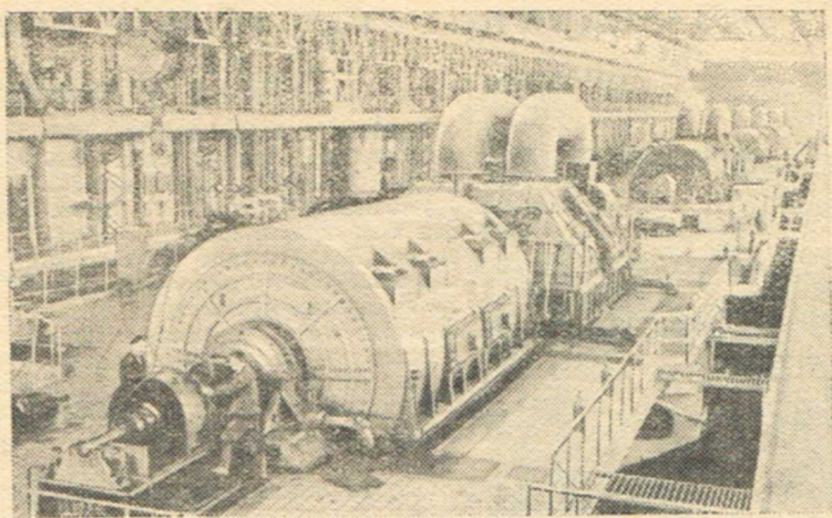
Сталинская область. На строительстве Славянской ГРЭС заканчивается монтаж турбины и двух котлов. Скоро мощность электростанции значительно возрастет.
