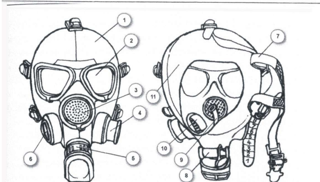
Рис. 26. Устройство гражданского противогаза ГП-9.
