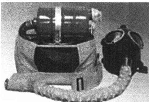
Рис. 33. Изолирующий противогаз ИП-4Р. Источник: Сайт ОАО «Сорбент» ( www.sorbent.su )
