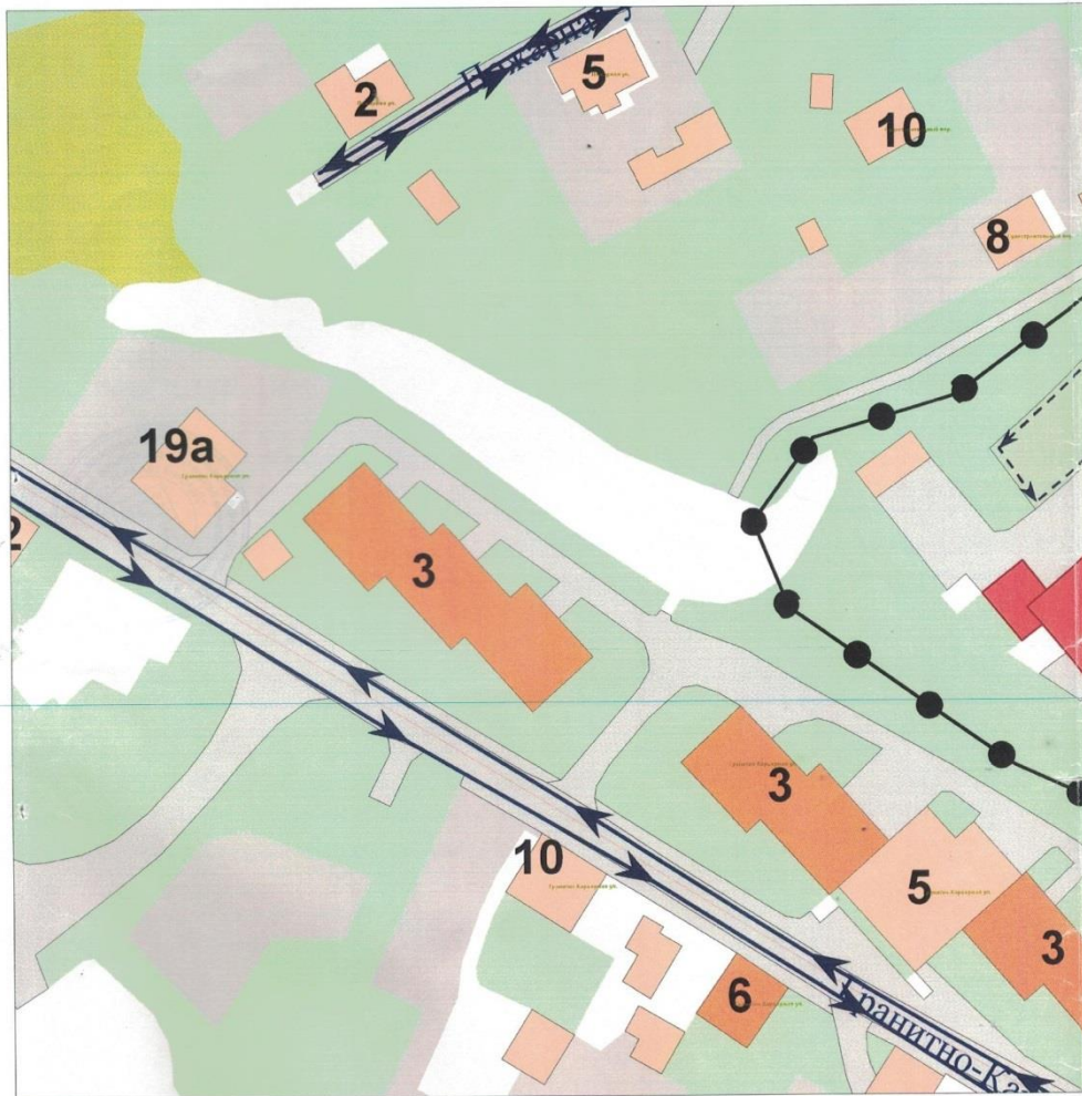
Пути движения транспортных средств и рекомендуемые пути передвижения детей по территории образовательного учреждения
