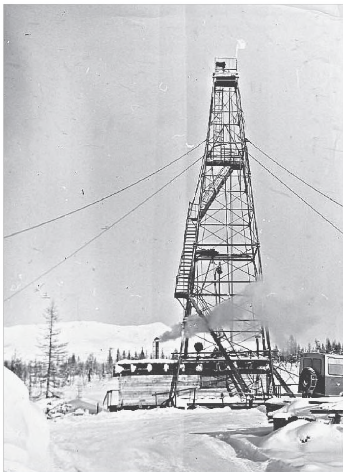
БУРОВАЯ ВЫШКА, ХОЛОДНИНСКОЕ ГЕОЛОГО-РАЗВЕДОЧНАЯ ПАРТИЯ 1983 ГОД
