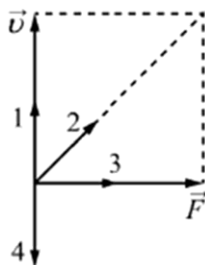
Рис. 2. Вектор скорости движущегося тела (материальной точки) и
