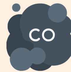
Отравление угарным газом
