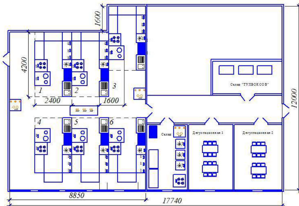
Общий план застройки рабочей площадки
