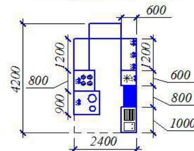
План рабочей зоны
