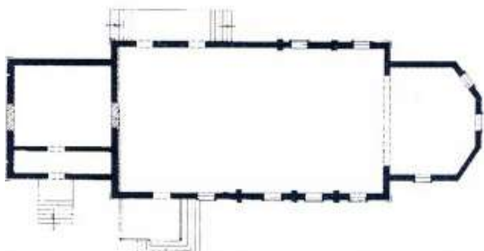
План Петропавловской церкви с. Быкова Чертеж 1989 г.
