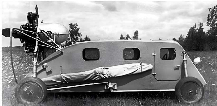
Аэросани НКЛ -16-42 на колесах
