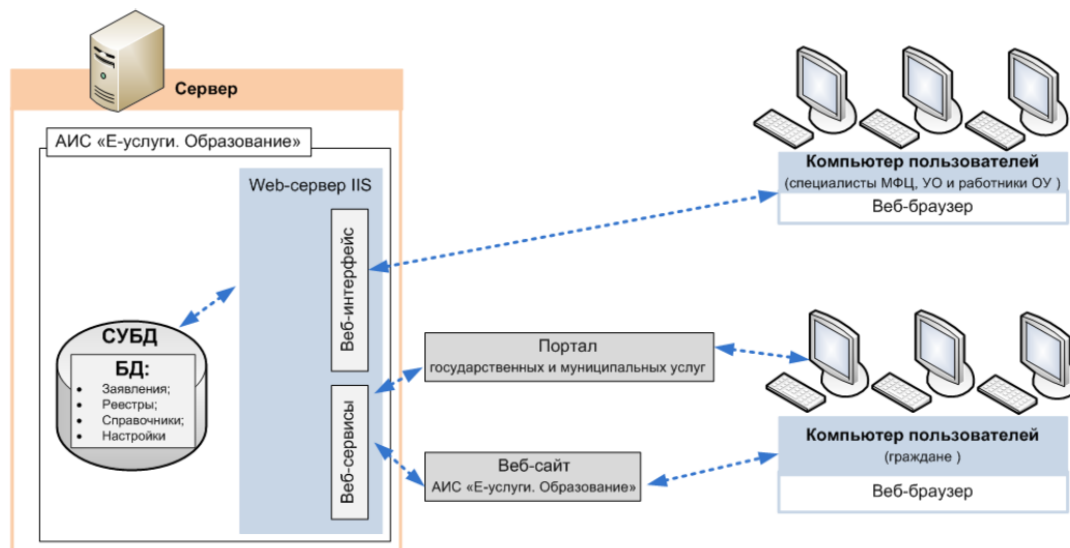
Рис.1 Общий вид технологического процесса ИСПДн.
