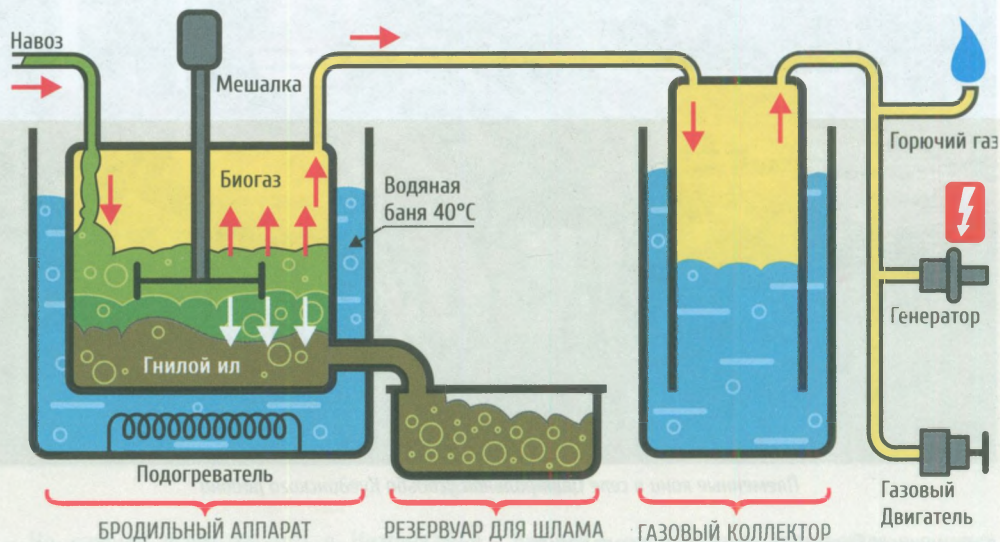
Принципиальная схема работы биогазовой установки
