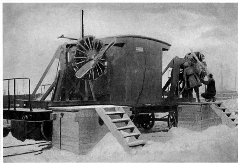
Авиационные моторы на испытаниях. Завод им. Сталина. 1940 г. ГАПО. Ф. р-1379. Оп. 1. Д. 108
