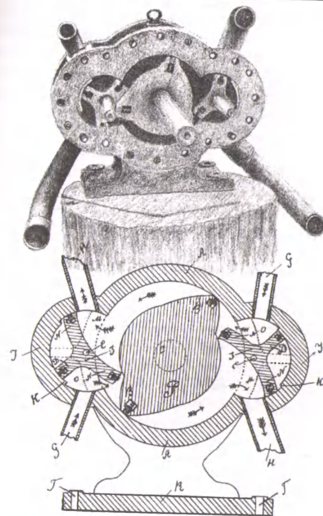
Изобретенный Г. И. Кобяком универсальный коловратно-ротаторный двигатель.
