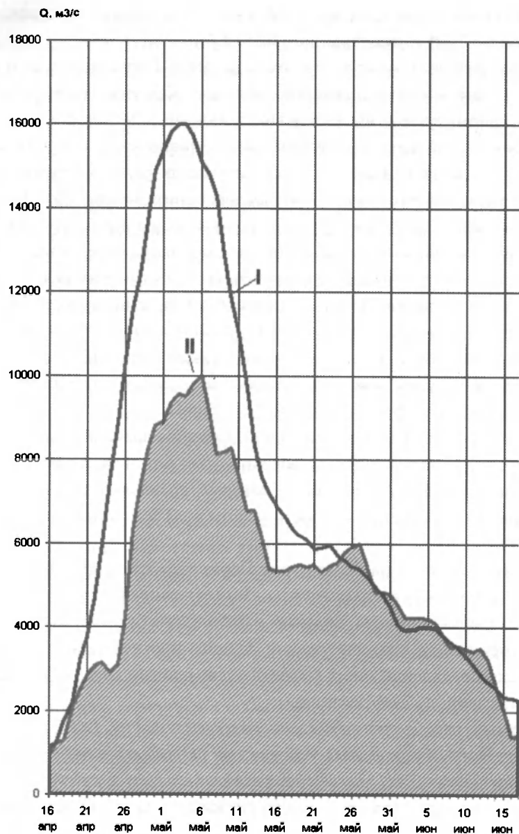
Рис. 4.1. Приток воды в Камское водохранилище (I) и сброс воды в створе ГЭС (II) в период половодья 2001 г.
