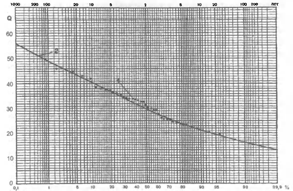
Рис. 4.2. Вероятность превышения (%) и повторяемости (лет) среднегодовых расходов воды ( Q \text{ м}^3/\text{с} ) реки Усьва у пос. Усьва: 1 – эмпирические данные, 2 – теоретическая кривая
