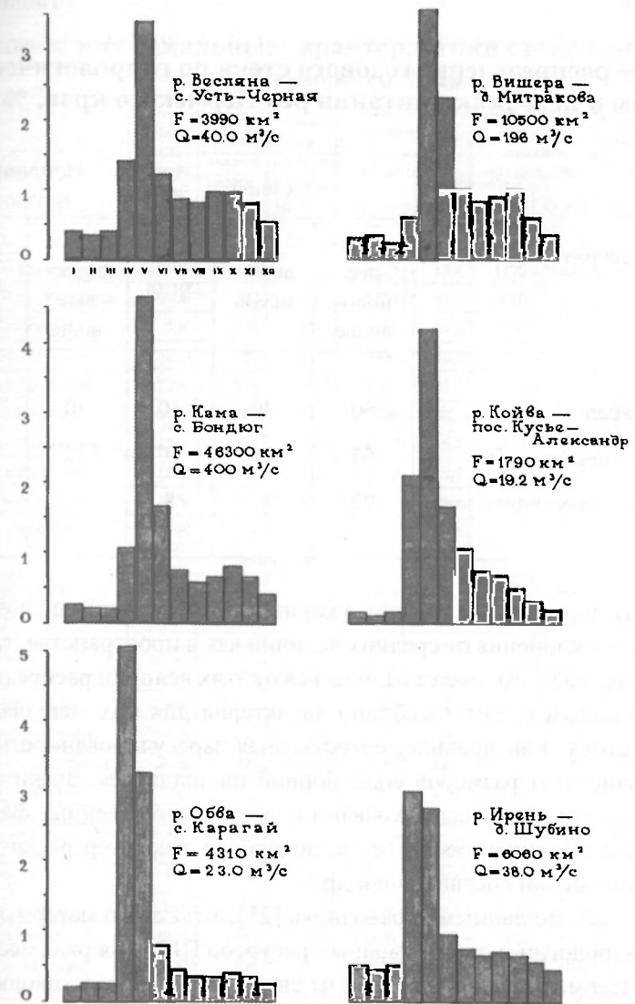
Рис. 2.2. Средние месячные расходы воды в долях от среднего годового:
