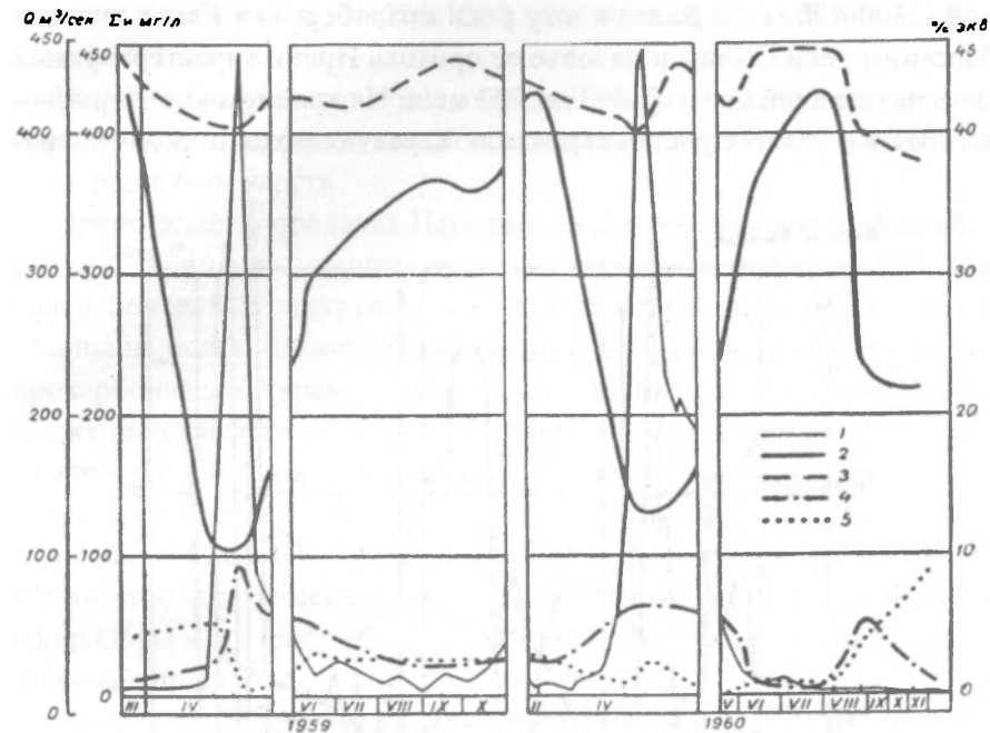
Рис. 6.2. Сезонное изменение минерализации и химического состава воды р. Обва у с. Карагай ( F=4310 \text{ км}^2 ): 1 – расход воды, Q \text{ м}^3/\text{с} ; 2 – сумма ионов \Sigma , мг/л; 3 – \text{HCO}_3^- ; 4 – \text{SO}_4^{2-} ; 5 – \text{Cl}^- , (% экв)
