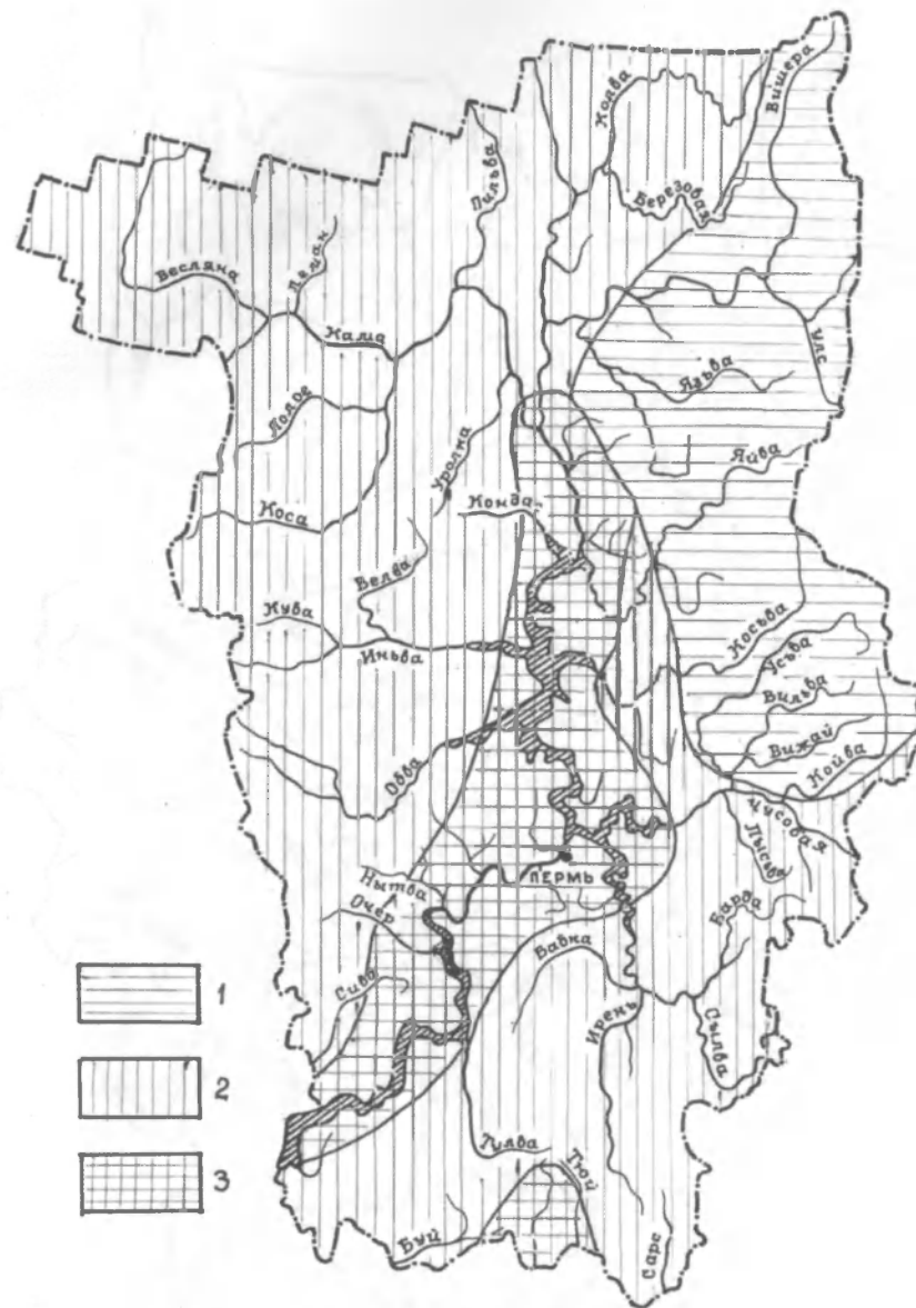
Рис. 6.4. Качество речных вод: 1 – хорошее, 2 – удовлетворительное, 3 – неудовлетворительное качество
