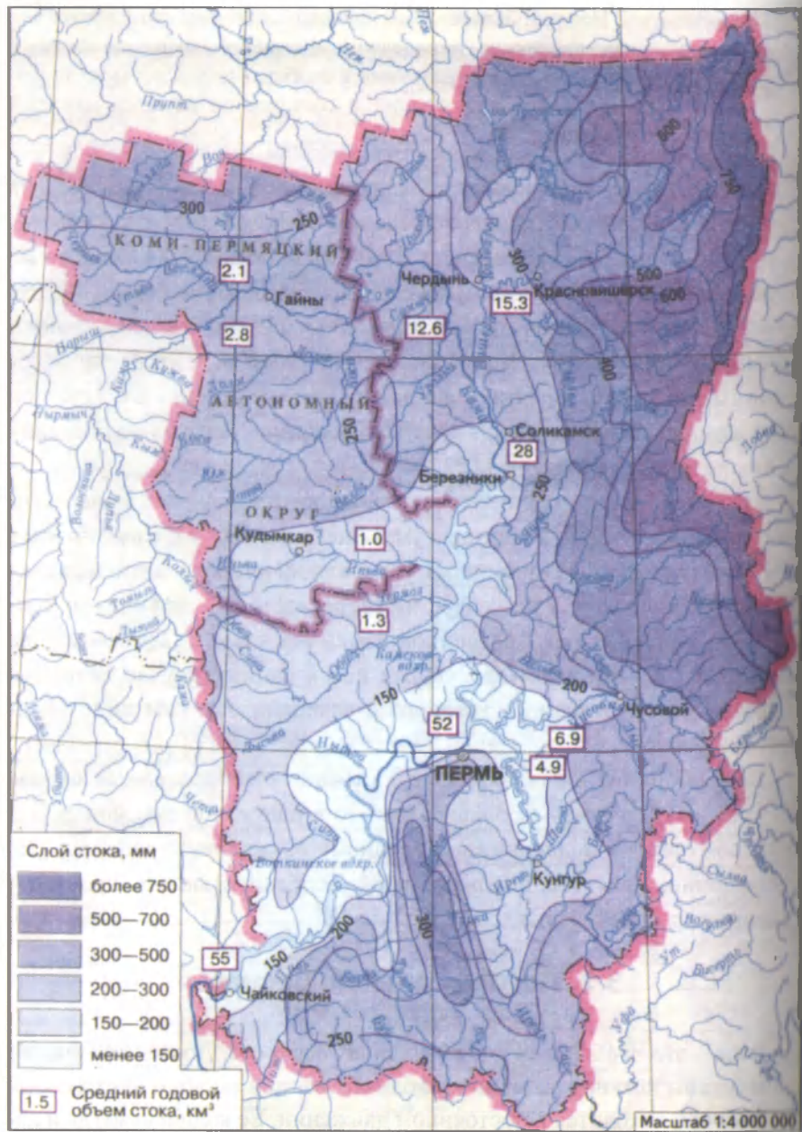
Рис. 3.1. Средний слой (мм) и объем (км 3 ) годового стока рек
