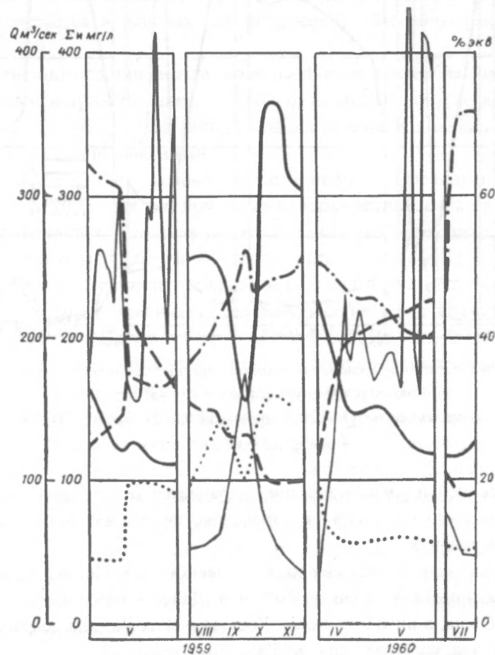
Рис. 6.3. Сезонное изменение минерализации ( \Sigma_n мг/л) и химического состава русловых вод пониженной минерализации, формирующихся на водосборе второй группы (р. Косьва – с. Останино, F=6220 км 2 ): 1 – расход воды, Q м 3 /с; 2 – сумма ионов \Sigma_n мг/л; 3 – \text{HCO}_3^- ; 4 – \text{SO}_4^{2-} ; 5 – \text{Cl}^- , (% экв)
