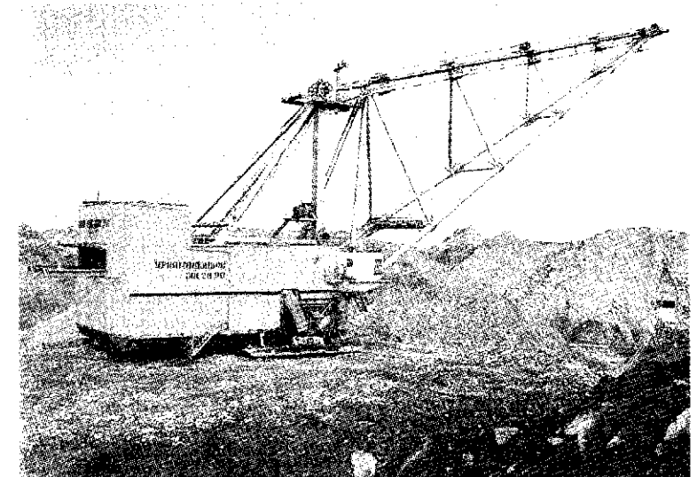
Уралмашевский богатырь — шагающий экскаватор с ковшом емкостью 20 кубометров и 90-метровой стрелой.
