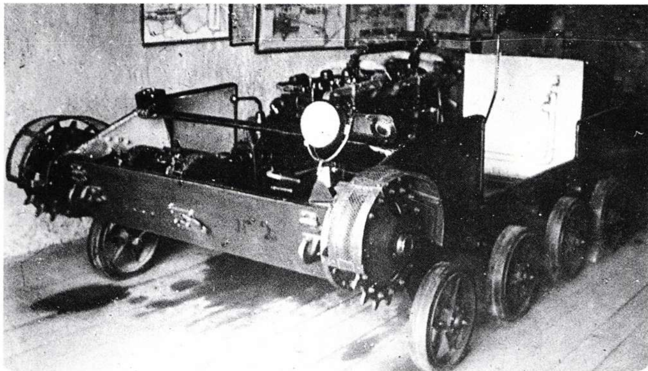
№ 71. Часть разобранного танка Т-34, установленная в одном из классов по изучению материальной части танков в Киевском танкотехническом училище. г. Кунгур, Молотовская область. 1943 г. КГА. Ф. 477. Оп. 1. Д. 289. Л. 19.
