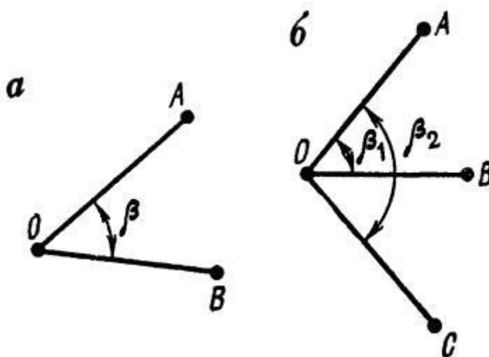
Рис. 1 Способы измерения горизонтальных углов: а - способ приемов; б - способ круговых приемов
