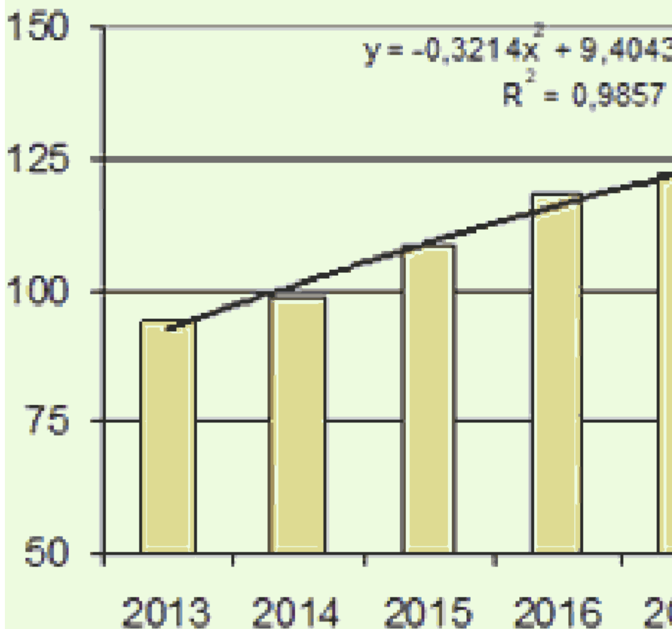
Рисунок 1 - Распространенность сахарного диабета у детей и подростков (на 100 тыс.)
