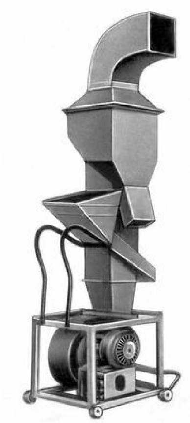
Пневматическая семяочистительная колонка ОПС-2Д-ОК
