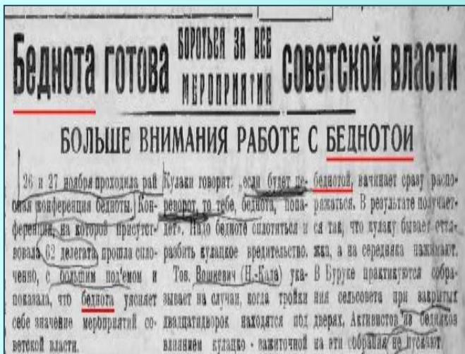
Собрание бедноты
