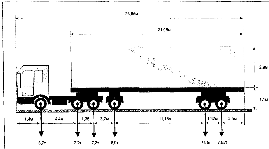
СХЕМА тяжеловесного и (или) крупногабаритного транспортного средства (автопоезда)
