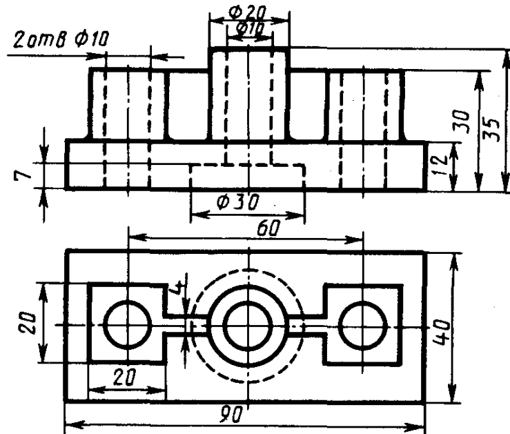
Опора
