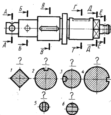
Рис. 8 Чертеж детали к упражнению 3.
