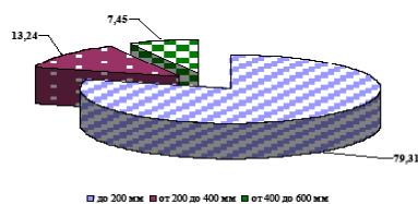
Рисунок 2.1.2.1. Структура тепловых сетей
