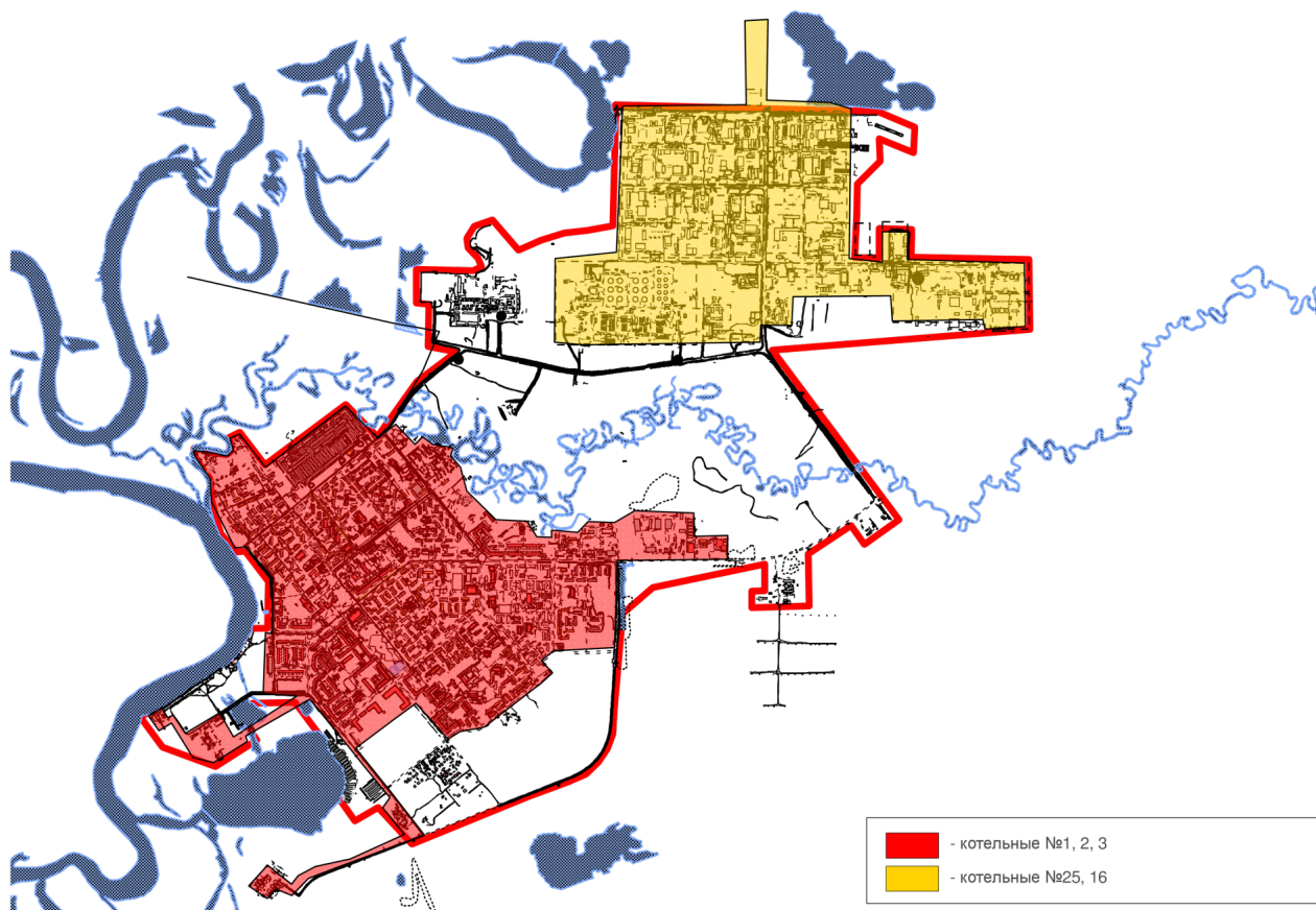
Рисунок 4 Зоны действия систем теплоснабжения и источников тепловой энергии
