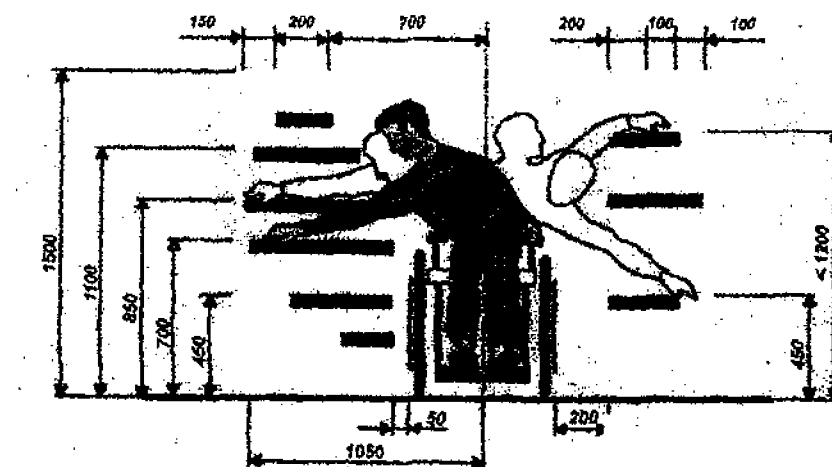
Рисунок Д.1. Кресло-коляска для взрослых
