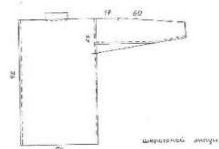
Ил. Схема крой верхней одежды.
