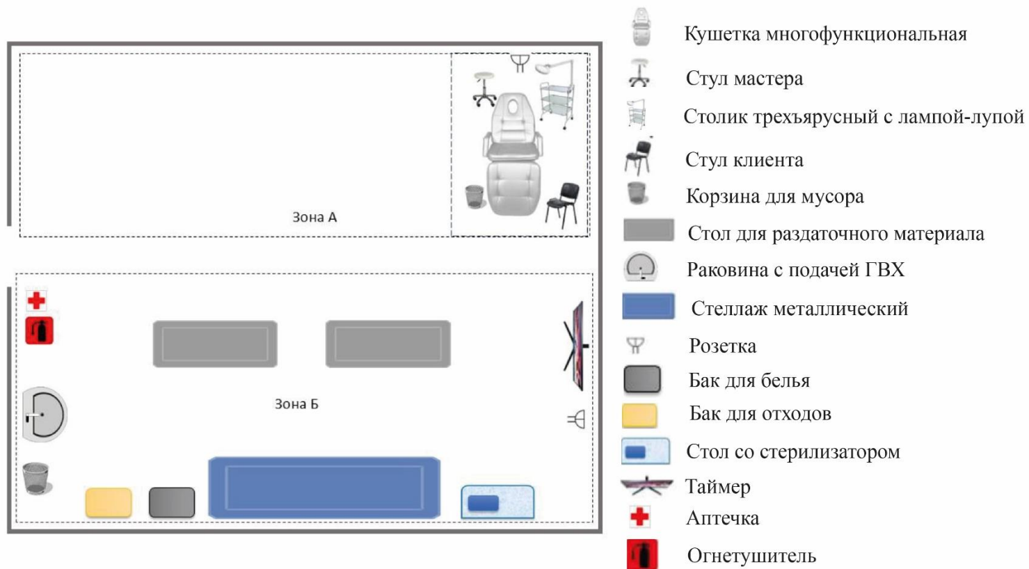
Рисунок 1 - План застройки площадки центра проведения демонстрационного экзамен
