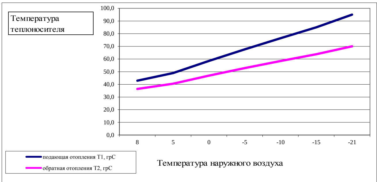
Температура наружного воздуха. °C Температура прямой сетевой воды, °C Температура обратной сетевой воды, °C 8 42,9 36,4 5 48,9 40,5 0 58,5 46,9 -5 67,6 52,8 -10 76,4 58,4 -15 85,0 63,8 -21 95,0 70,0
