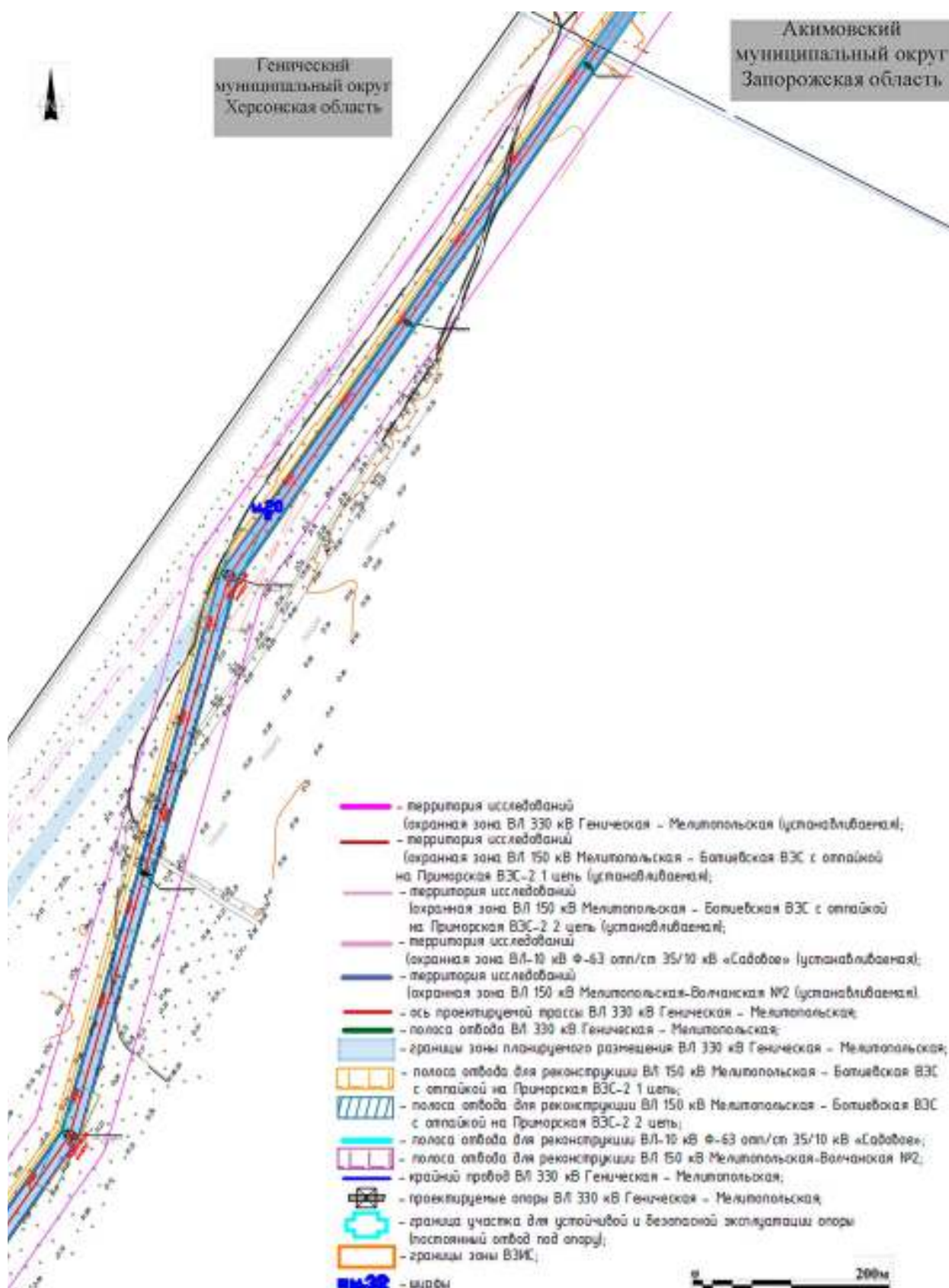
Рис. 65. Херсонская область. Строительство ВЛ 330 кВ Геничеськая - Мелитопольская. Схема расположения территории исследований и разведочных шурфа 20 на топографическом плане Заказчика. Лист 33.
