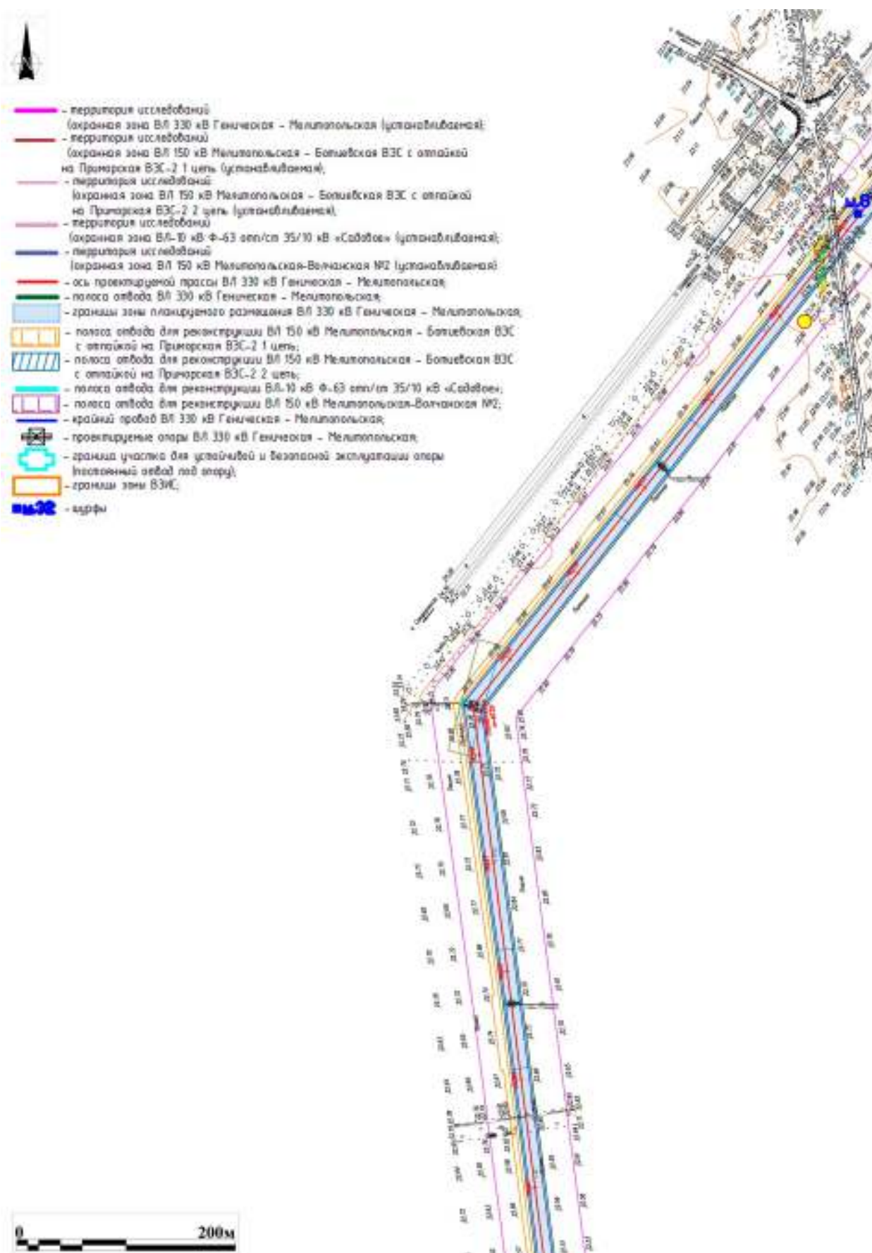
Рис. 55. Херсонская область. Строительство ВЛ 330 кВ Геническая - Мелитопольская. Схема расположения территории исследований и разведочного шурфа 8 на топографическом плане Заказчика. Лист 23.
