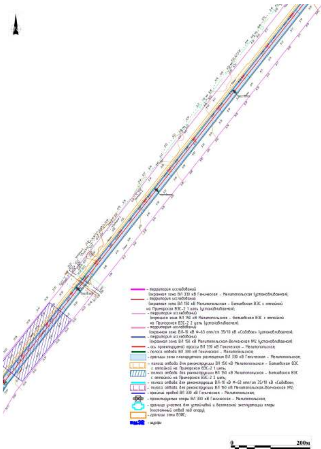
Рис. 34. Херсонская область. Строительство ВЛ 330 кВ Геническая - Мелитопольская. Схема расположения территории исследований на топографическом плане Закачка.
