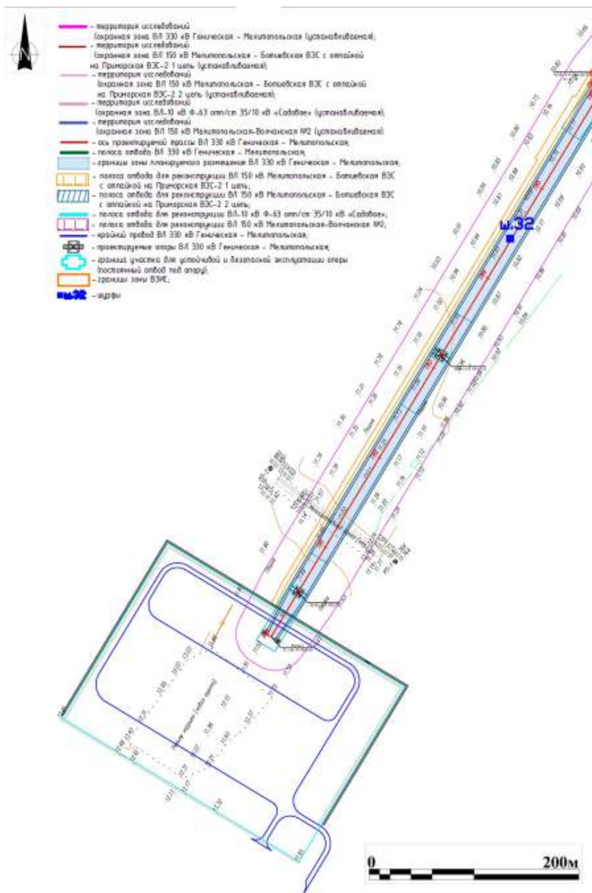
Рис. 33. Херсонская область. Строительство ВЛ 330 кВ Геническая - Мелитопольская. Схема расположения территории исследований и разведочного шурфа 32 на топографическом плане Заказчика. Лист 1.
