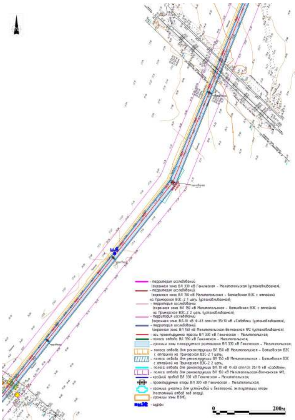
Рис. 43. Херсонская область. Строительство ВЛ 330 кВ Геническая - Мелитопольская. Схема расположения территории исследований и разведочного шурфа 6 на топографическом плане Заказчика. Лист 11.
