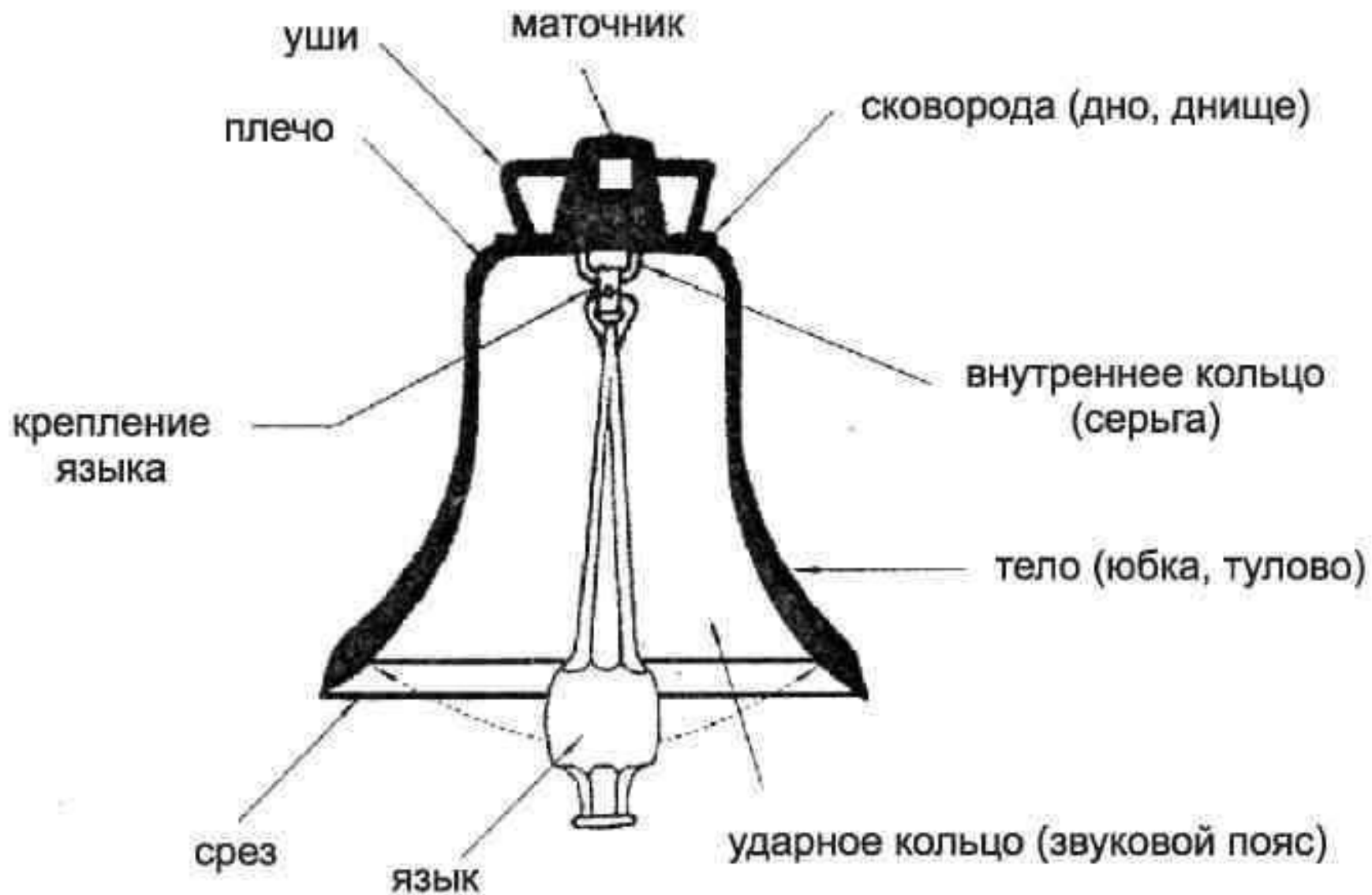
Примерный вид колокола и его основные части
