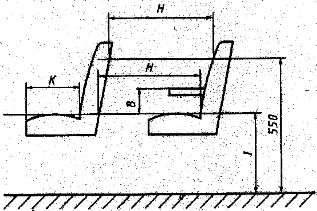
Рисунок 1.16.1. Размеры и расположение сидений
